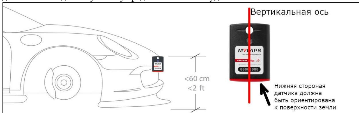
Рисунок 1. Схема монтажа датчика хронометража.
